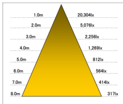
■直下照度及び配光曲線
