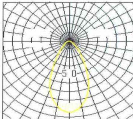
配光曲線 cd/1000LM
