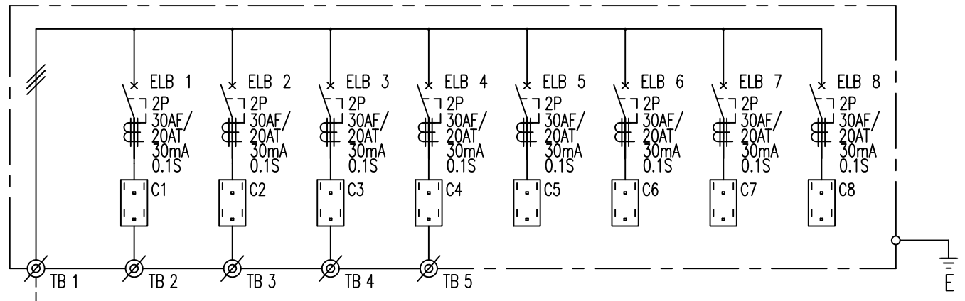
結線図
