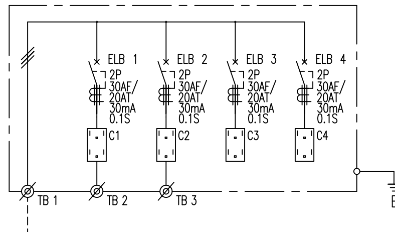
結線図
