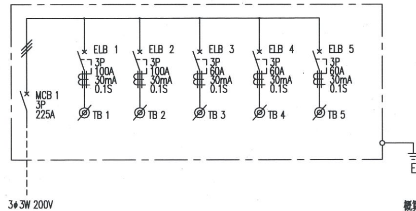
結線図
