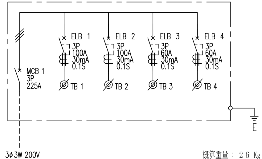
結線図
