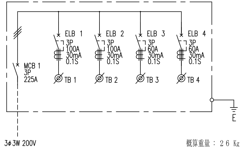
結線図
