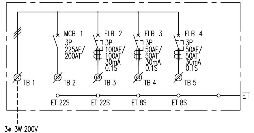
結線図
