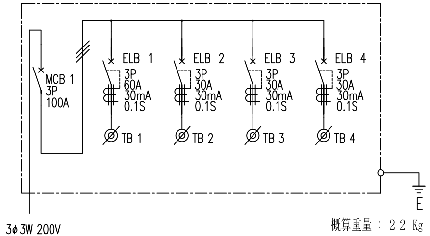
結線図
