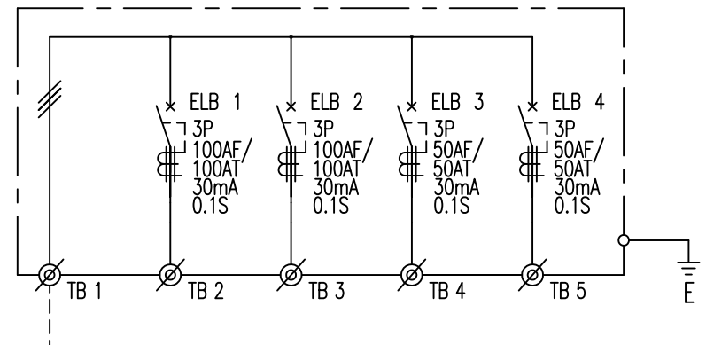
結線図
