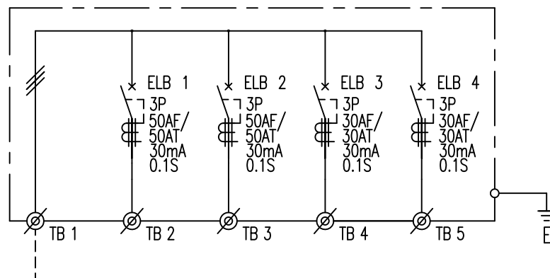
結線図
