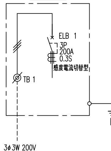
結線図
