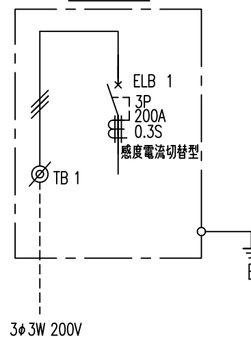
結線図
