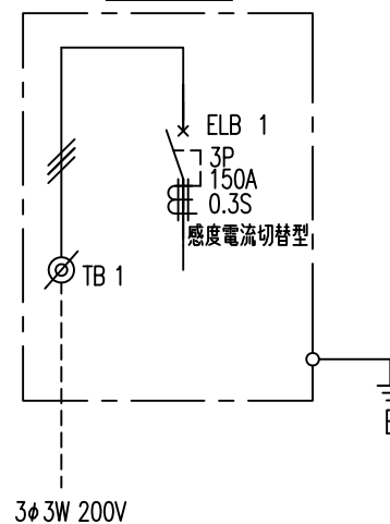
結線図
