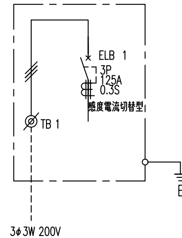
結線図
