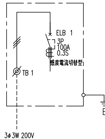
結線図
