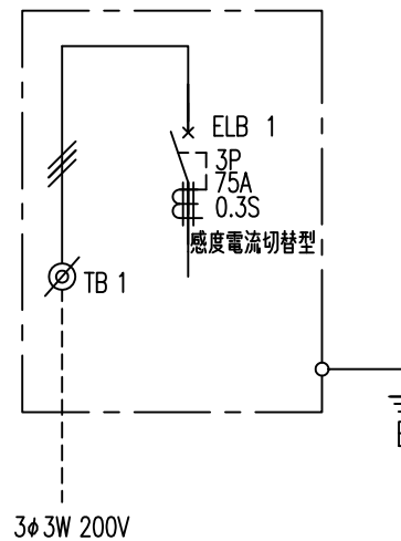
結線図
