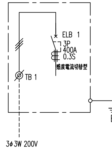
結線図
