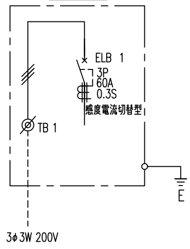
結線図
