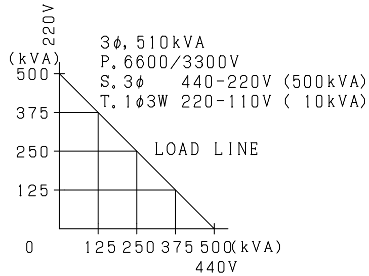
負荷分担図
